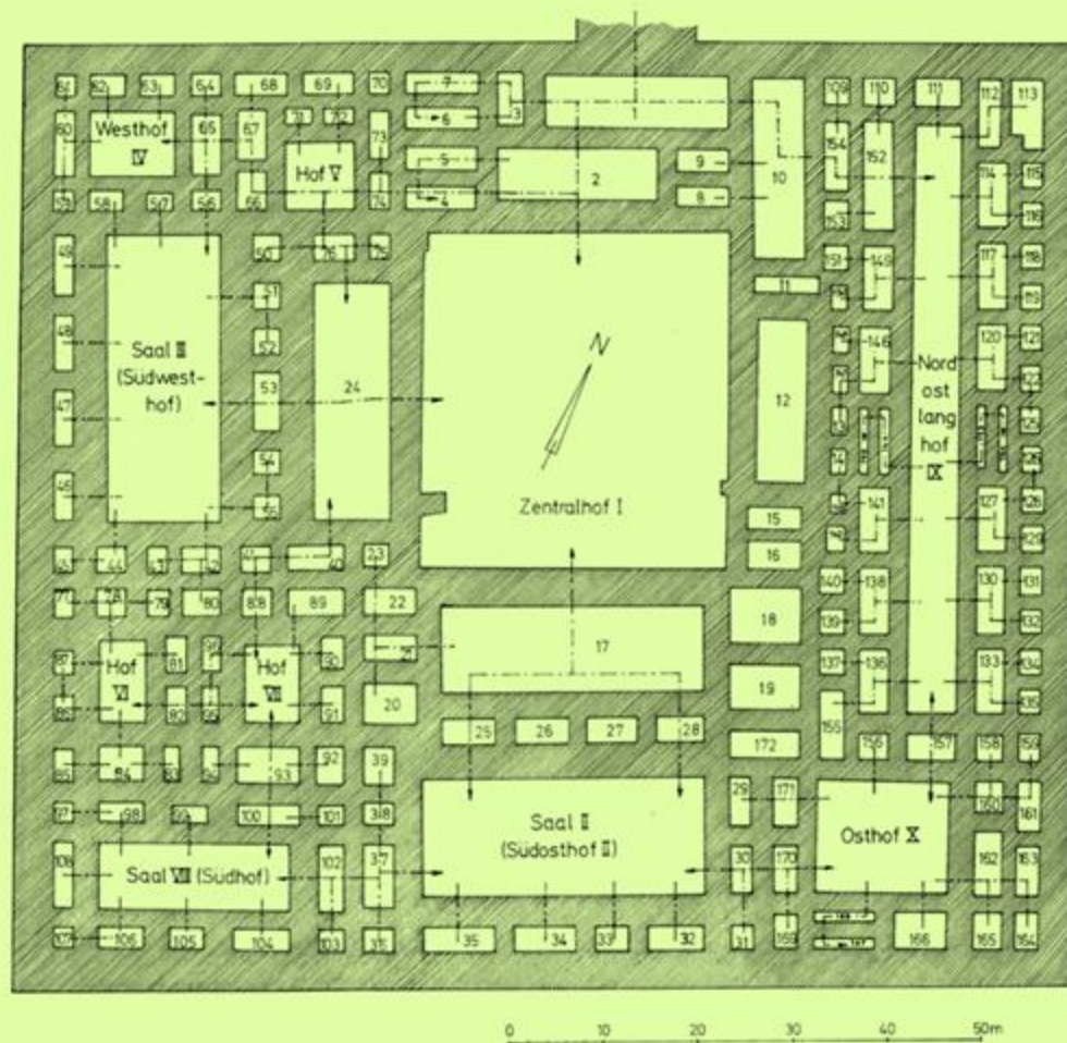
Fig. 44 Assur: palazzo vecchio (1:1000) (Preusser 1955, tav. 3; Heinrich 1984, fig. 24).
